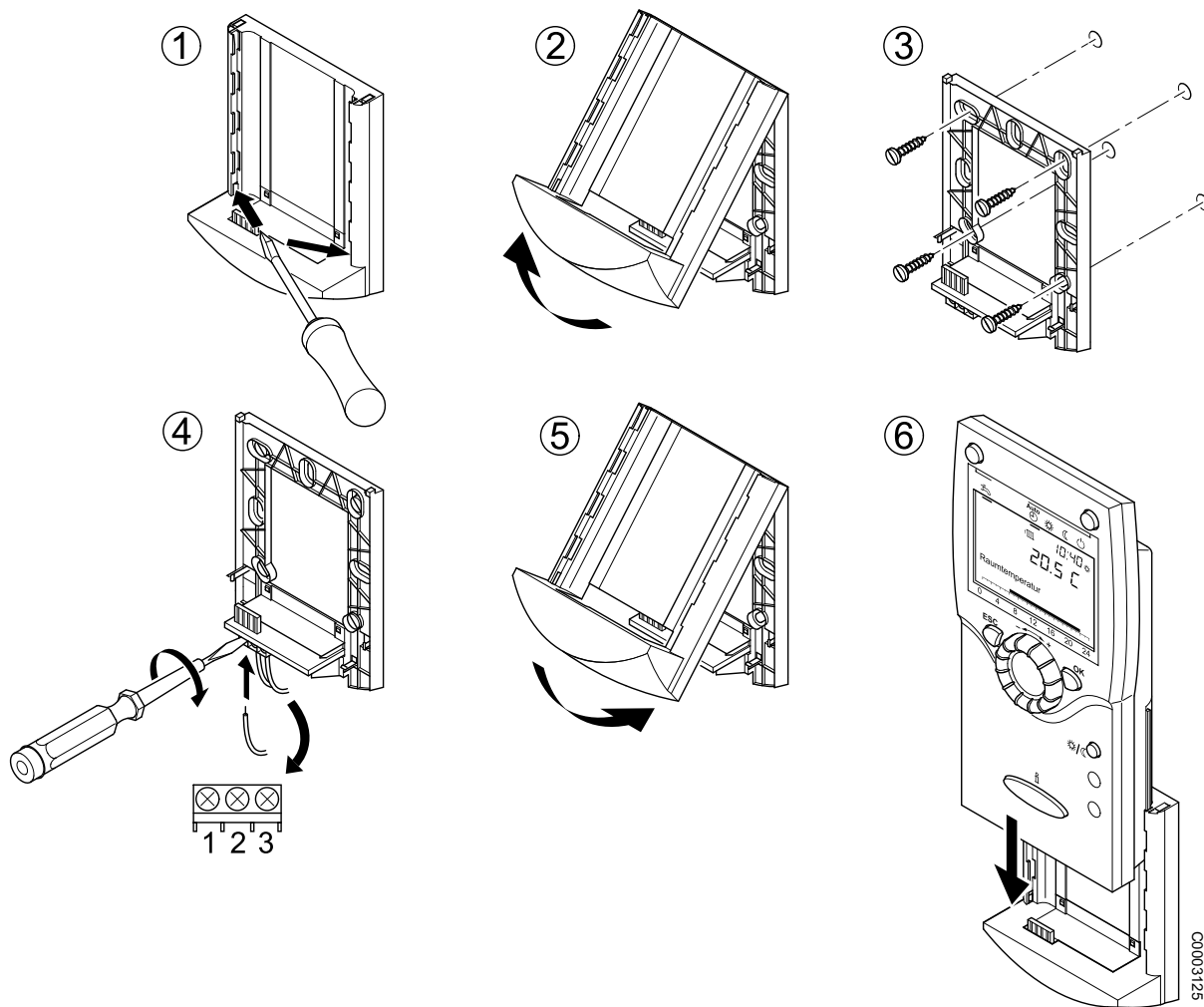
Rys. 6: Montaż regulatora pokojowego RGT/RGTK
