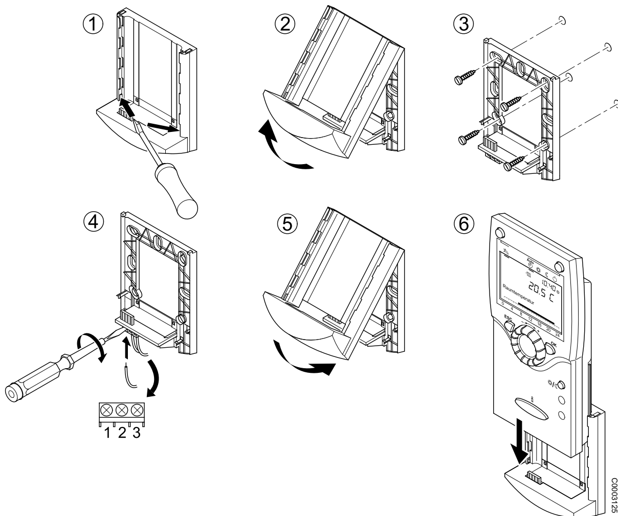
Ábra. 6: RGT/RGTK szobatermosztát szerelése
