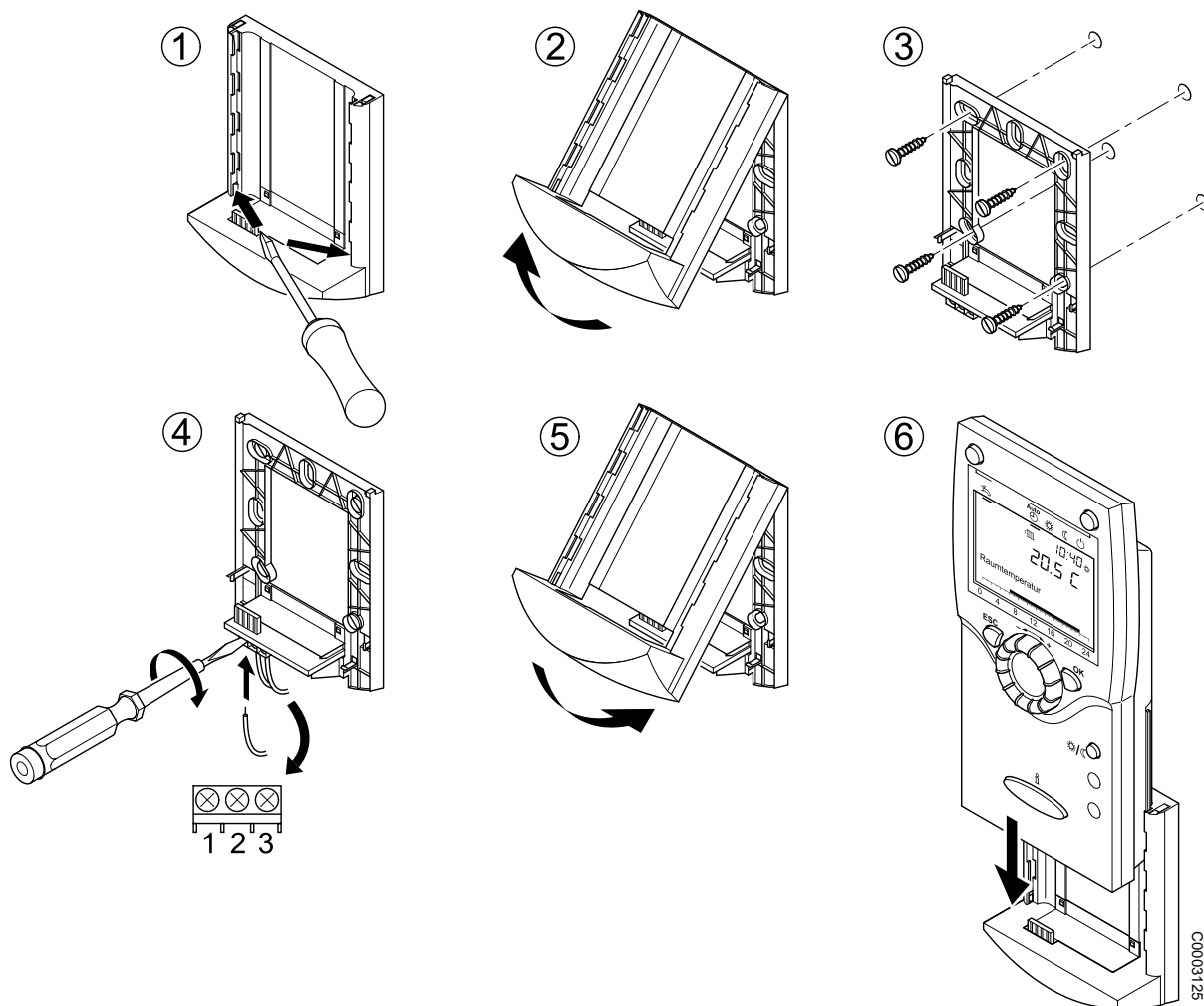
Abb. 6: Montage des Raumgerätes RGT/RGTK
