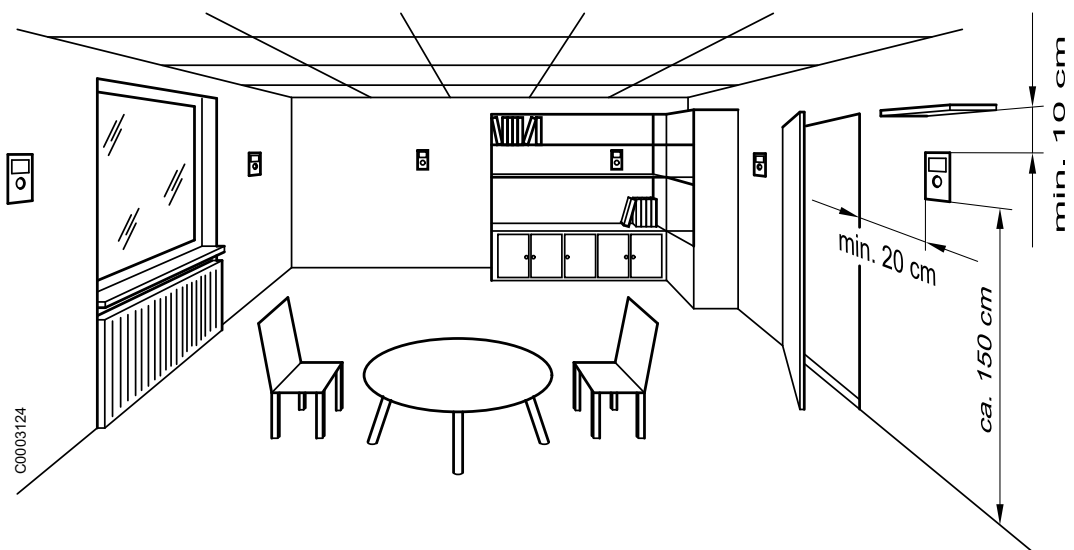
Rys. 5: Miejsce zamontowania regulatora (przykłady montażu)
