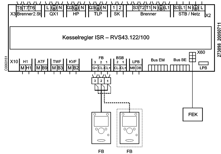
Abb. 2: Schaltplan für Anschluss an Systemregler ISR-RVS
