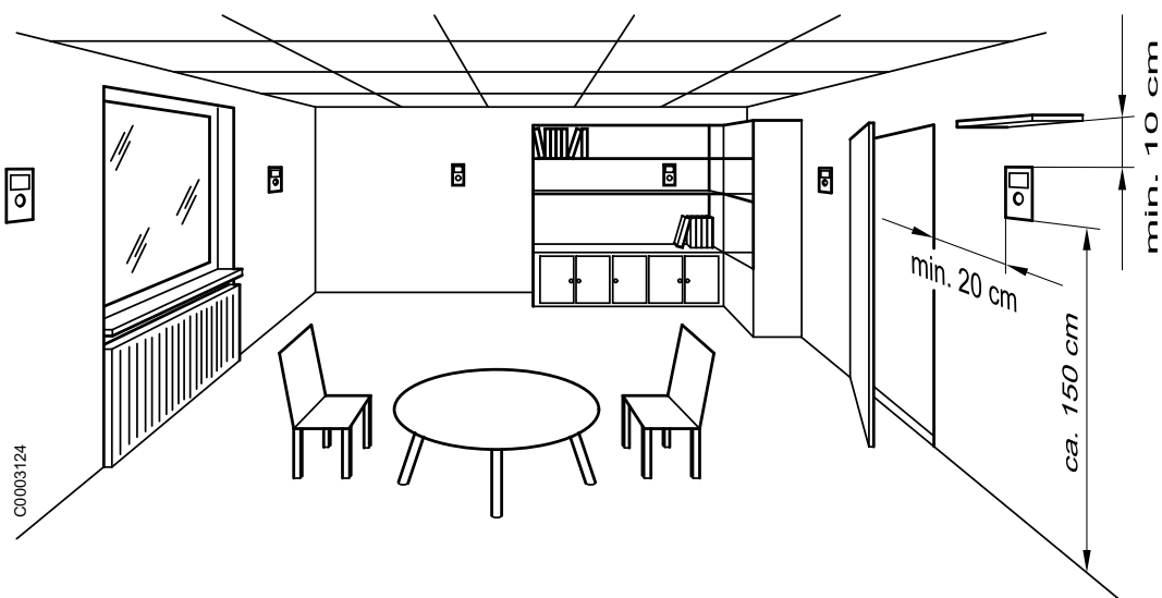
Fig. 5: Monteringssted (eksempler på montering)
