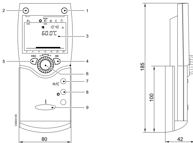
Afb. 1: Overzicht en Afmetingen
