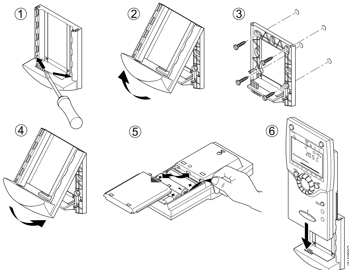
Rys. 7: Montaż regulatora pokojowego RGTF/RGTKF
