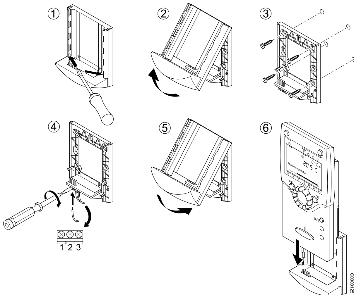
Afb. 6: Montage van de ruimte unit RGT/RGTK
