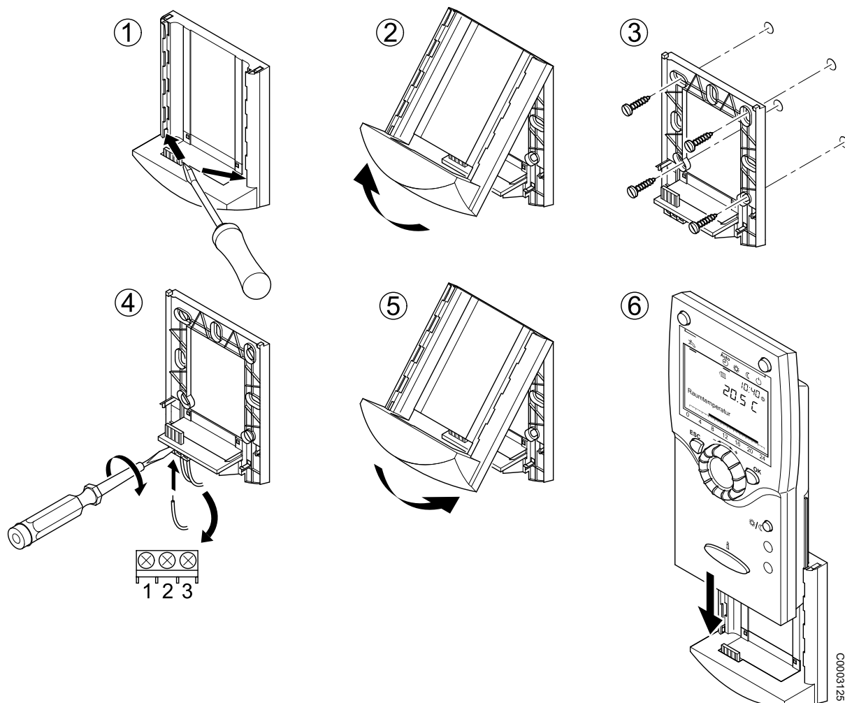
Obr. 6: Montáž termostatu RGT/RGTK
