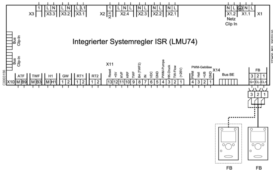
Afb. 3: Aansluitplan voor aansluiting aan de systeemregelaar ISR-LMU (vanaf LMU 74)
