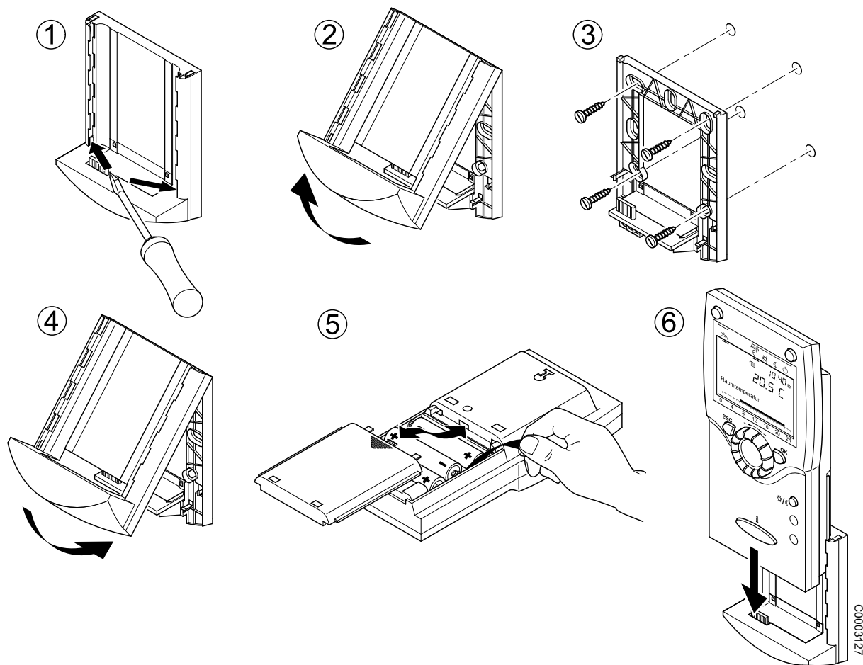
Obr. 7: Montáž termostatu RGTF/RGTKF
