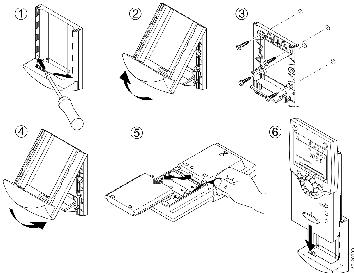
Abb. 7: Montage des Raumgerätes RGTF/RGTKF
