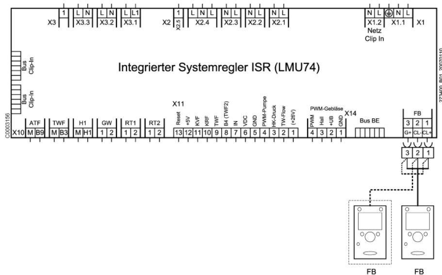
Ábra. 3: Kapcsolási vázlat az ISR-LMU rendszerszabályozóra való bekötéshez (az LMU 74-től)
