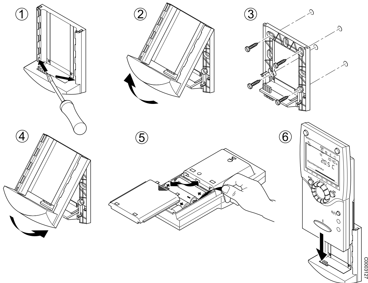
Afb. 7: Montage van de ruimte unit RGTF/RGTKF
