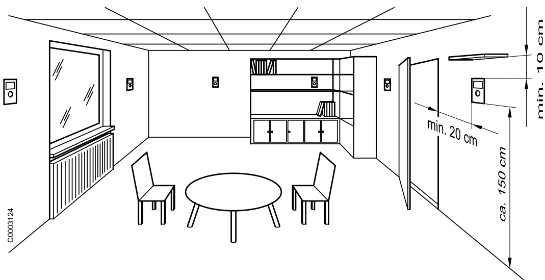
Obr. 5: Místo montáže (příklady montáže)
