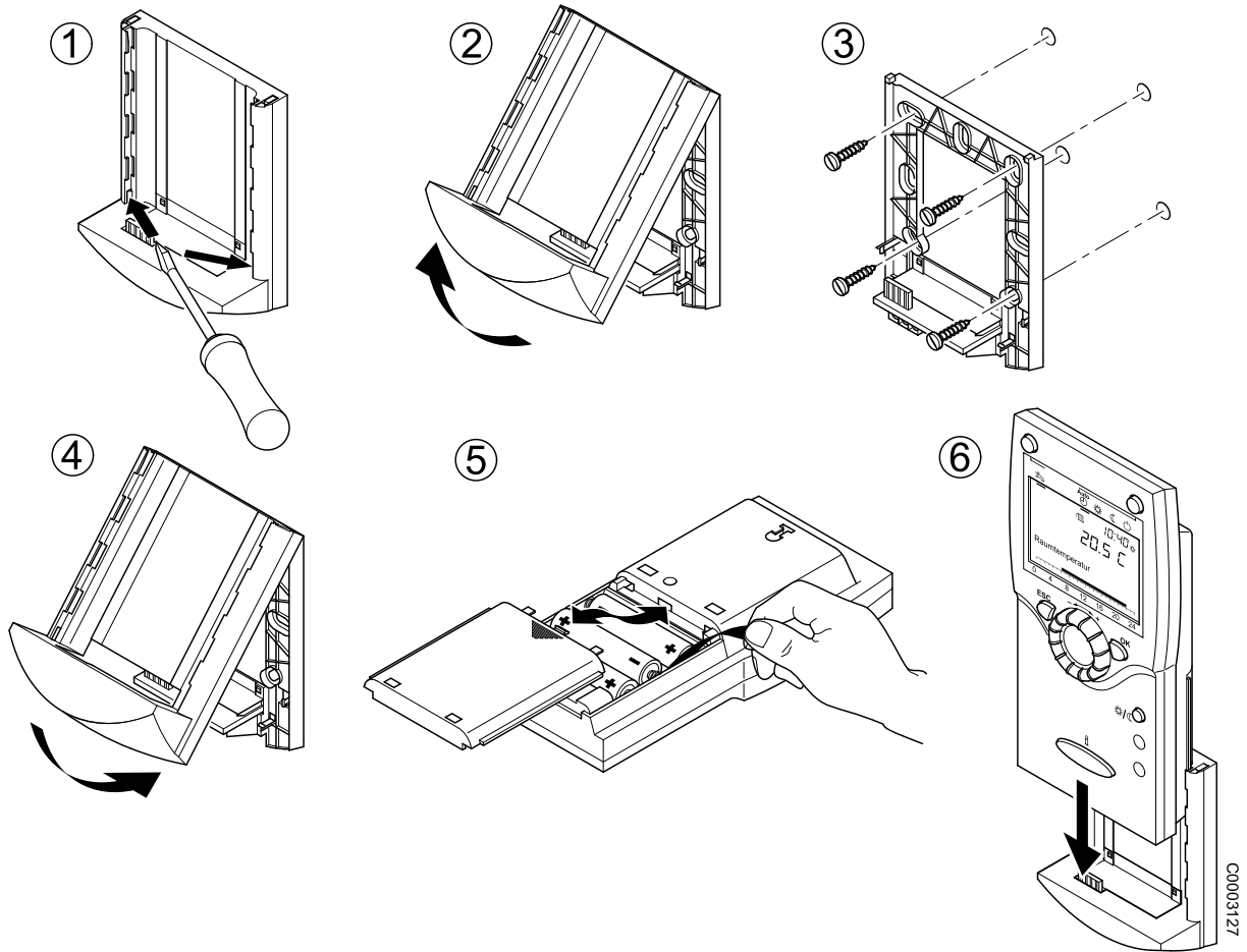
Ábra. 7: RGTF/RGTFK szobatermosztát szerelése
