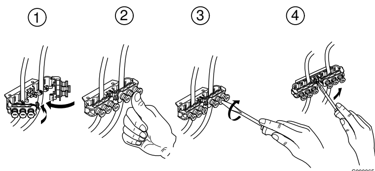
Obr. 10: Prvek odlehčení tahového pnutí
