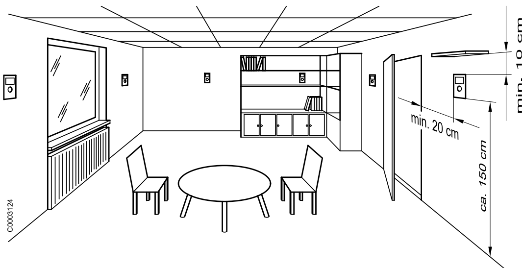
Fig 5: Lieu de montage (exemples d'installation)
