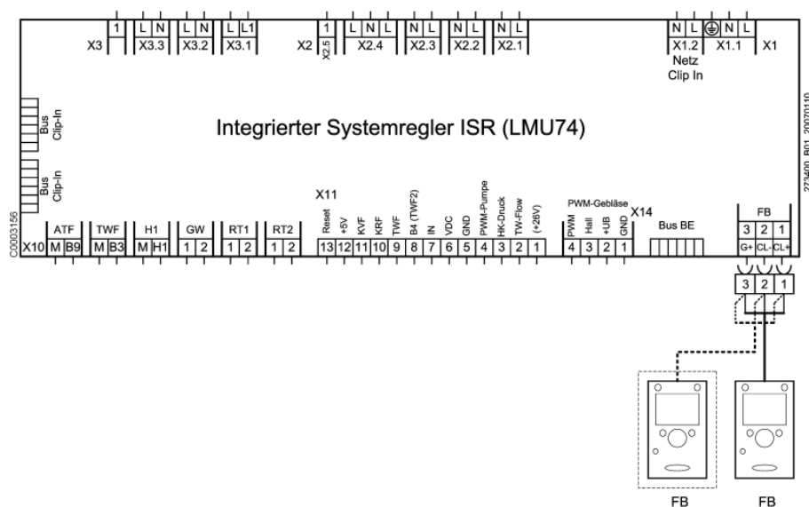
Rys. 3: Schemat podłączenia elektrycznego do regulatora systemowego ISR-LMU (w wersji od LMU 74)
