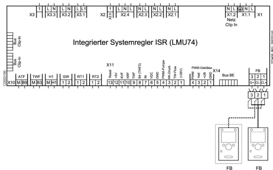
Abb. 3: Schaltplan für Anschluss an Systemregler ISR-LMU (ab LMU 74)
