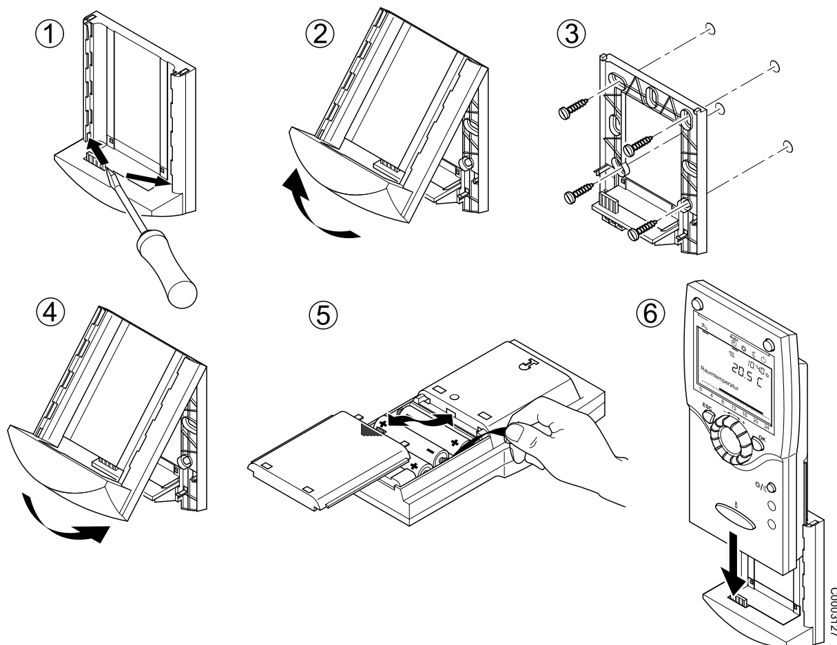
Fig. 7: Montering af RGTF/RGTKF-rumenhed
